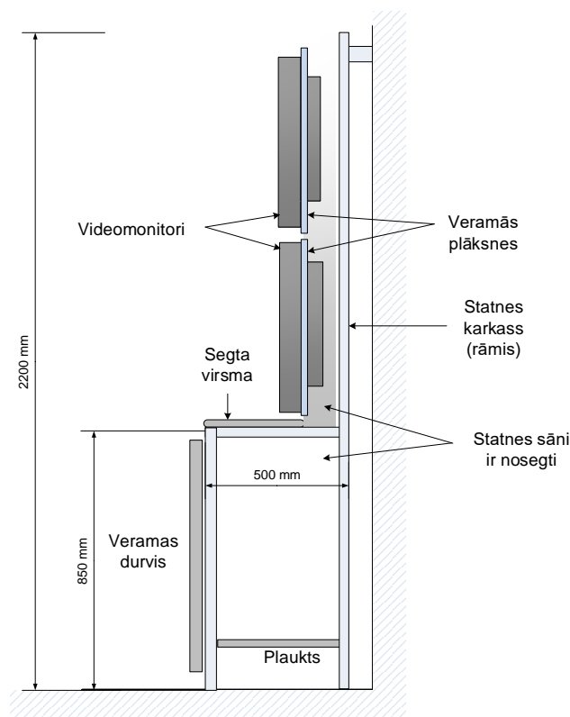
3. attēls. Statnes sānskata skice.
