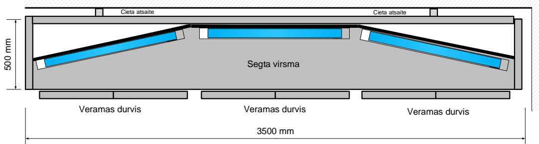
2. attēls. Statnes virsskata skice.
