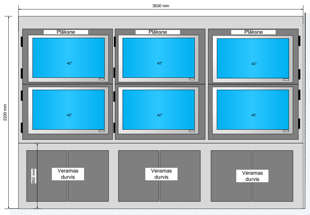
1. attēls. Statnes pretskata skice.
