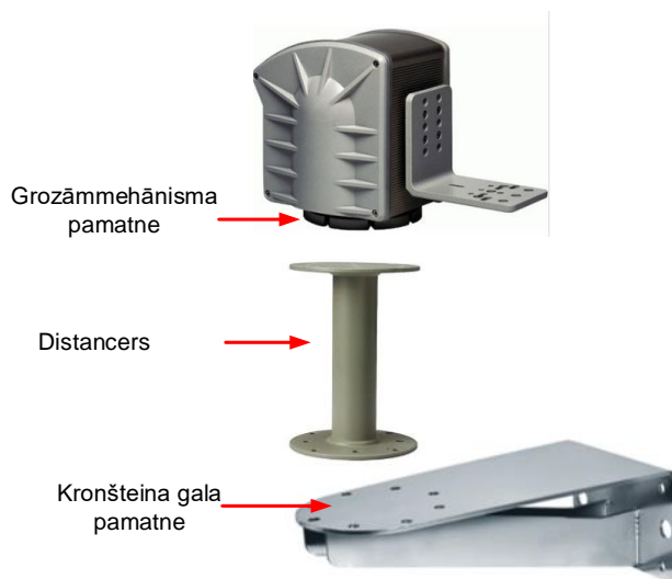
2. ilustratīvais attēls. Grozāmās videokameras kronšteina komponenti.
