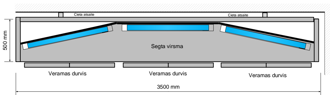
2. attēls. Statnes virsskata skice.
